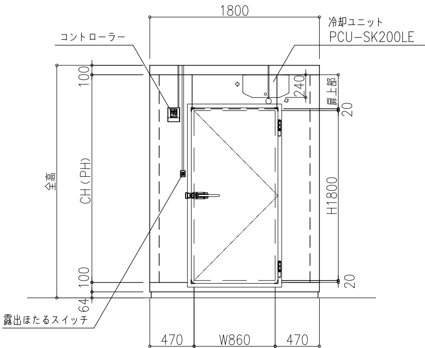
正面図 S=1/40
