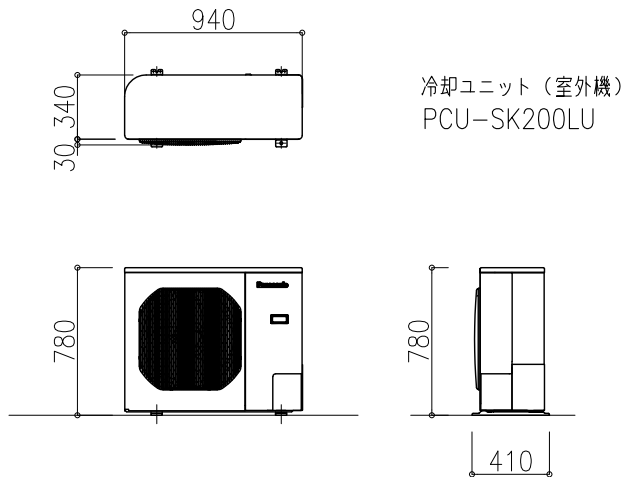
冷凍機姿図 S=1/40
