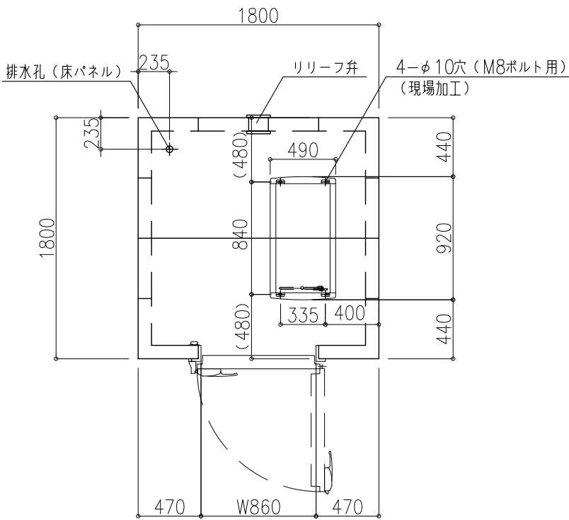
平面図 S=1/40
