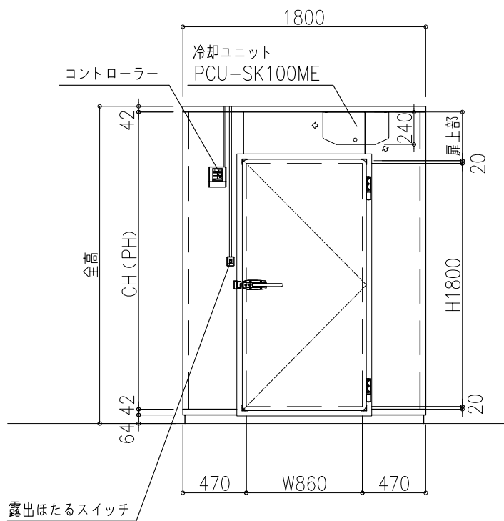
正面図 S=1/40
