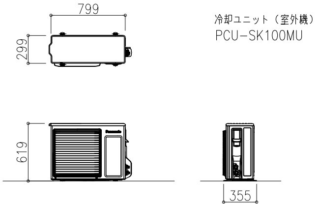
冷凍機姿図 S=1/40
