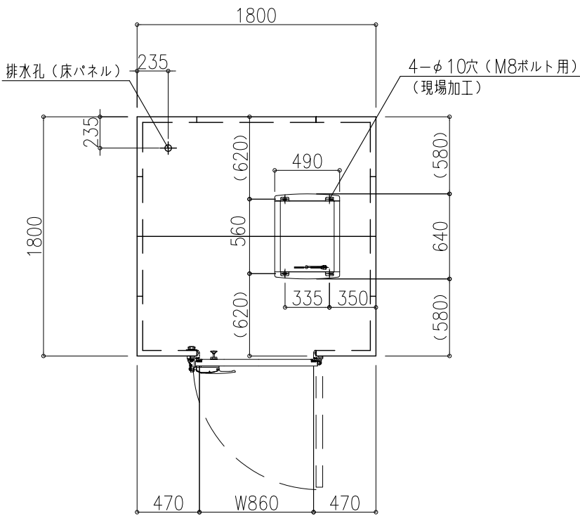
平面図 S=1/40
